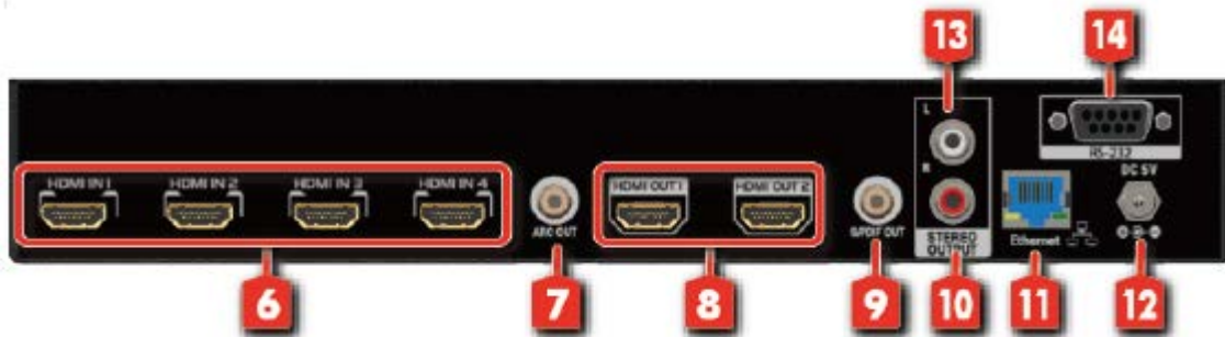
[図 3.2] リアパネルの外観図
